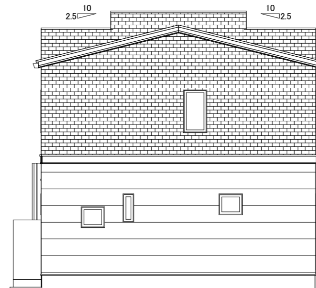
西側 立面図
