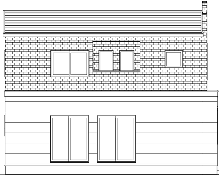
南側 立面図
