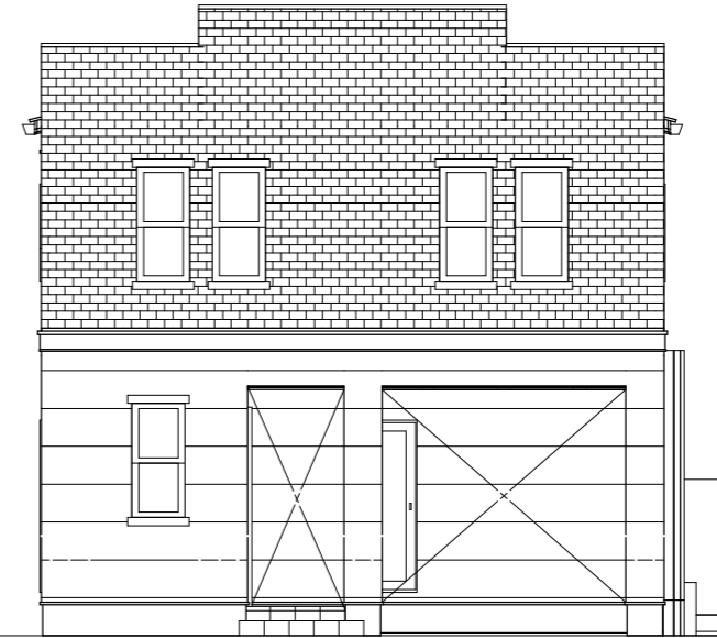
東側 立面図
