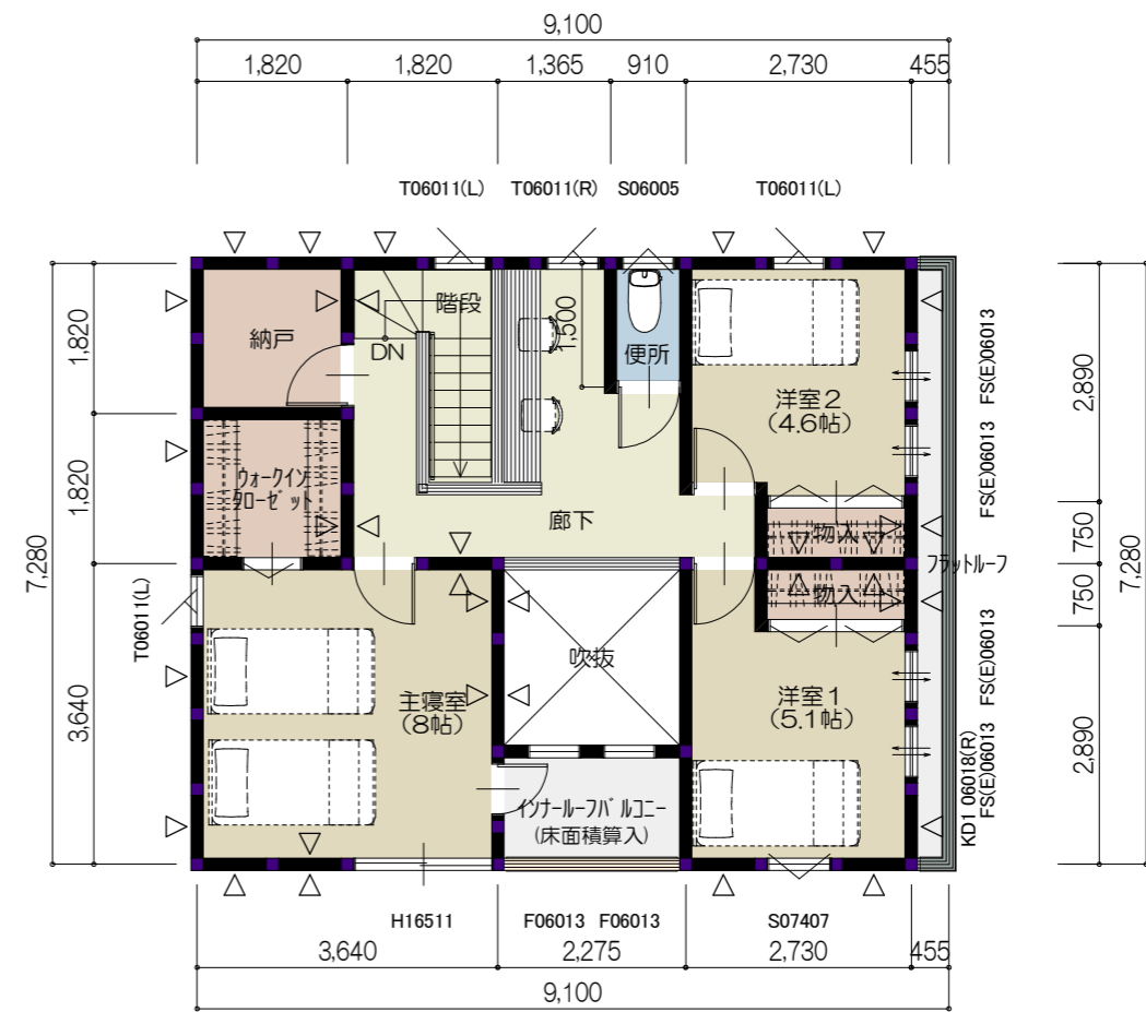
2階平面図
